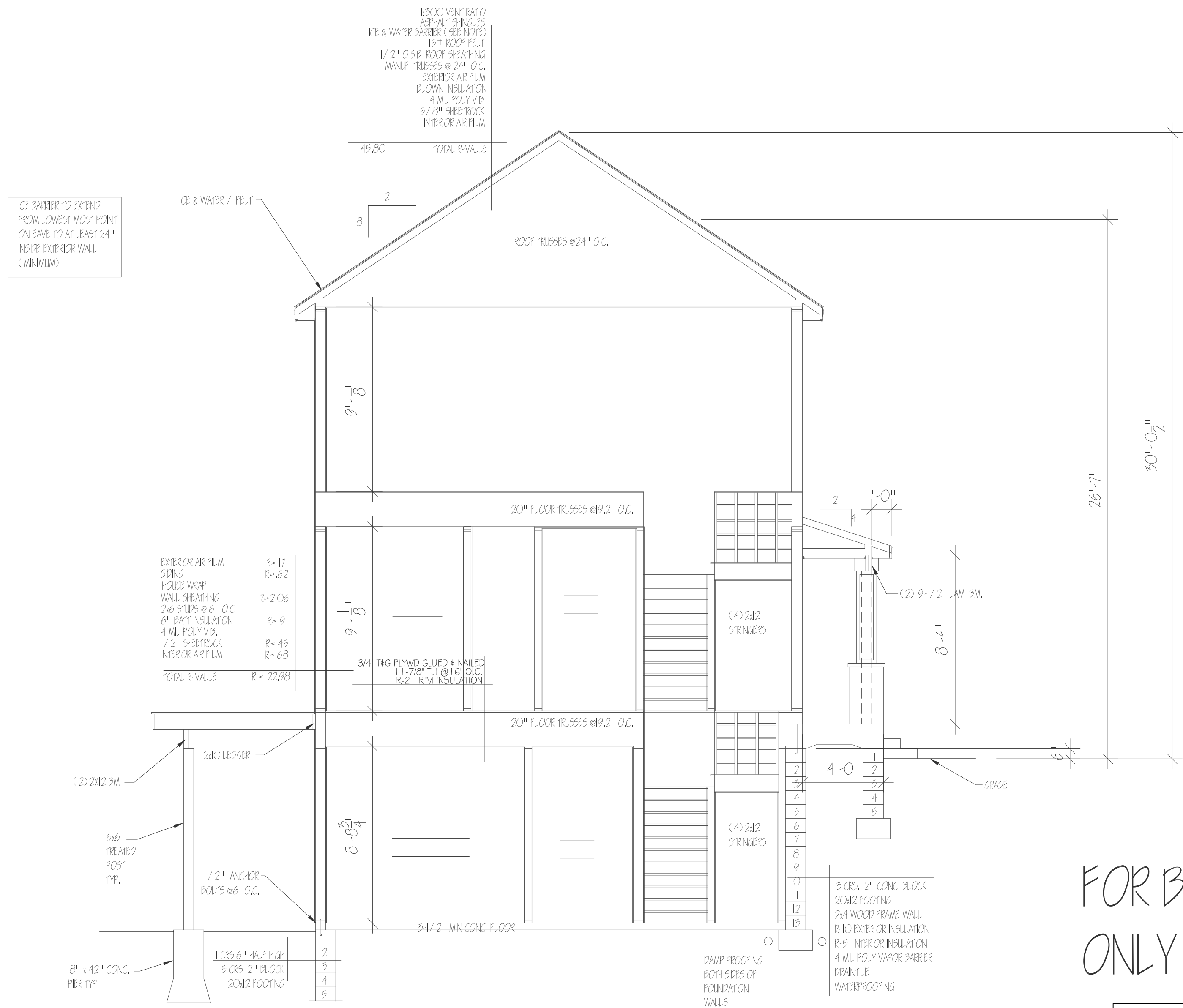
SECTION SCALE: 1/4" = 1'-0"
